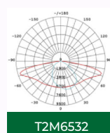
CURVA TII-M
